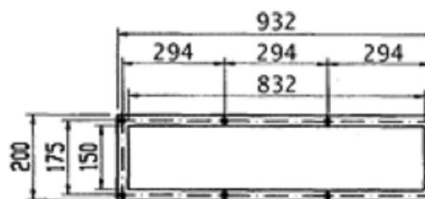
FLANGIA SCARICO FERRO
